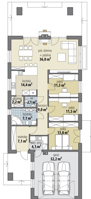
RZUT PARTER
