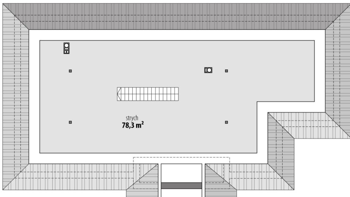
RZUT
