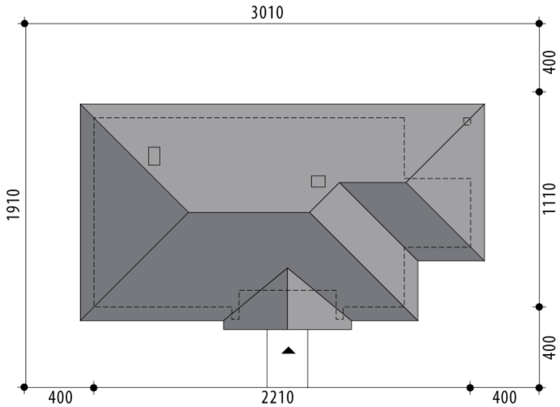
RZUT DZIAŁKI
