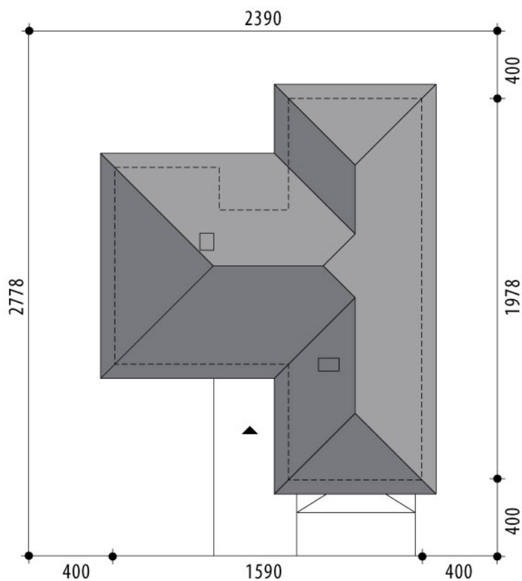
RZUT DZIAŁKI
