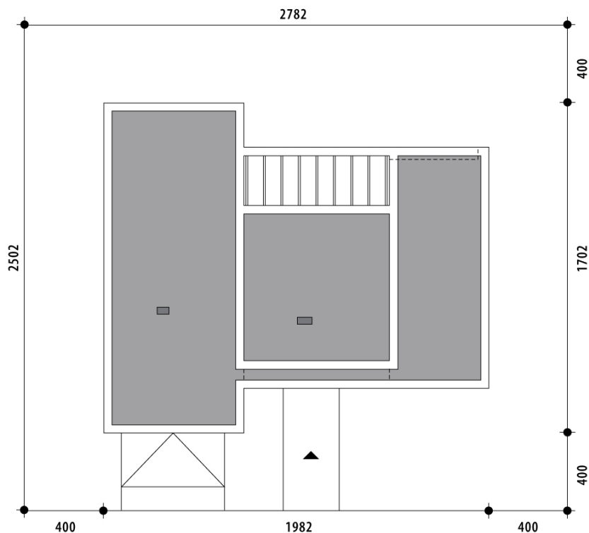
RZUT DZIAŁKI
