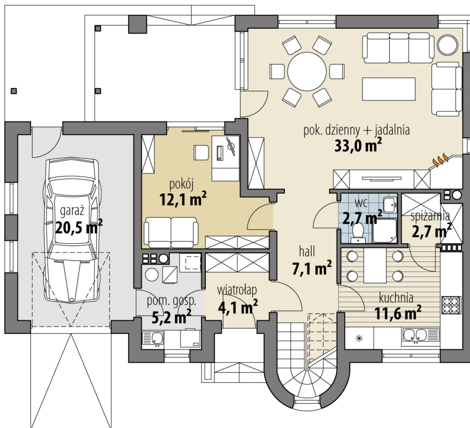
RZUT PARTER
