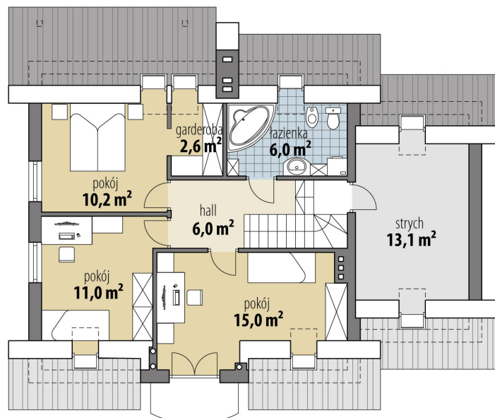
RZUT
