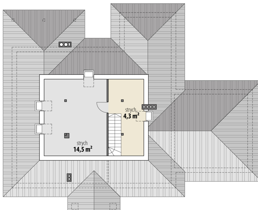
RZUT
