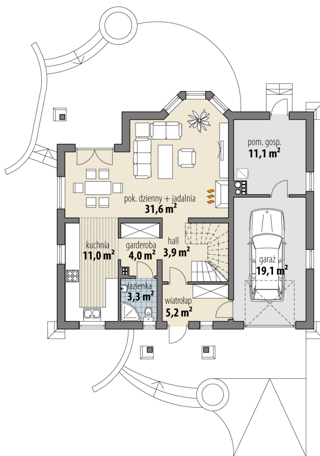
RZUT PARTER
