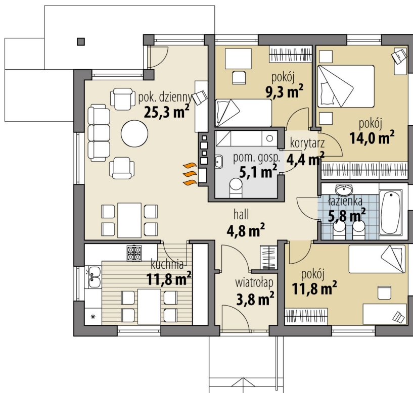
RZUT PARTER
