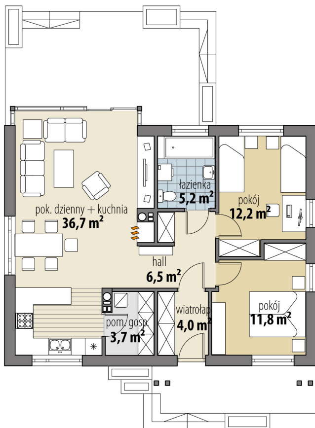
RZUT PARTER
