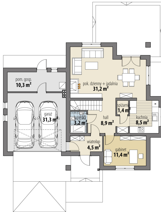
RZUT PARTER
