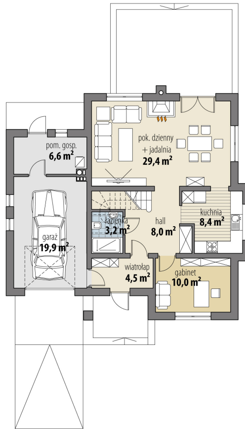
RZUT PARTER
