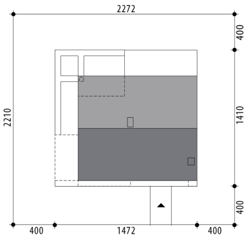
RZUT DZIAŁKI
