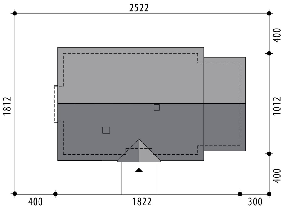
RZUT DZIAŁKI
