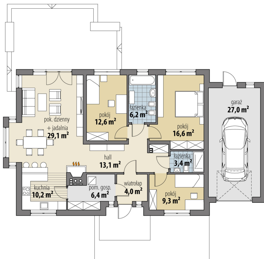
RZUT PARTER
