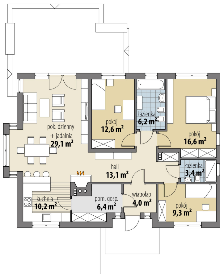
RZUT PARTER
