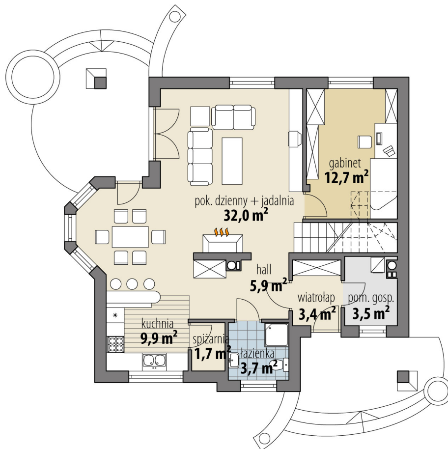
RZUT PARTER
