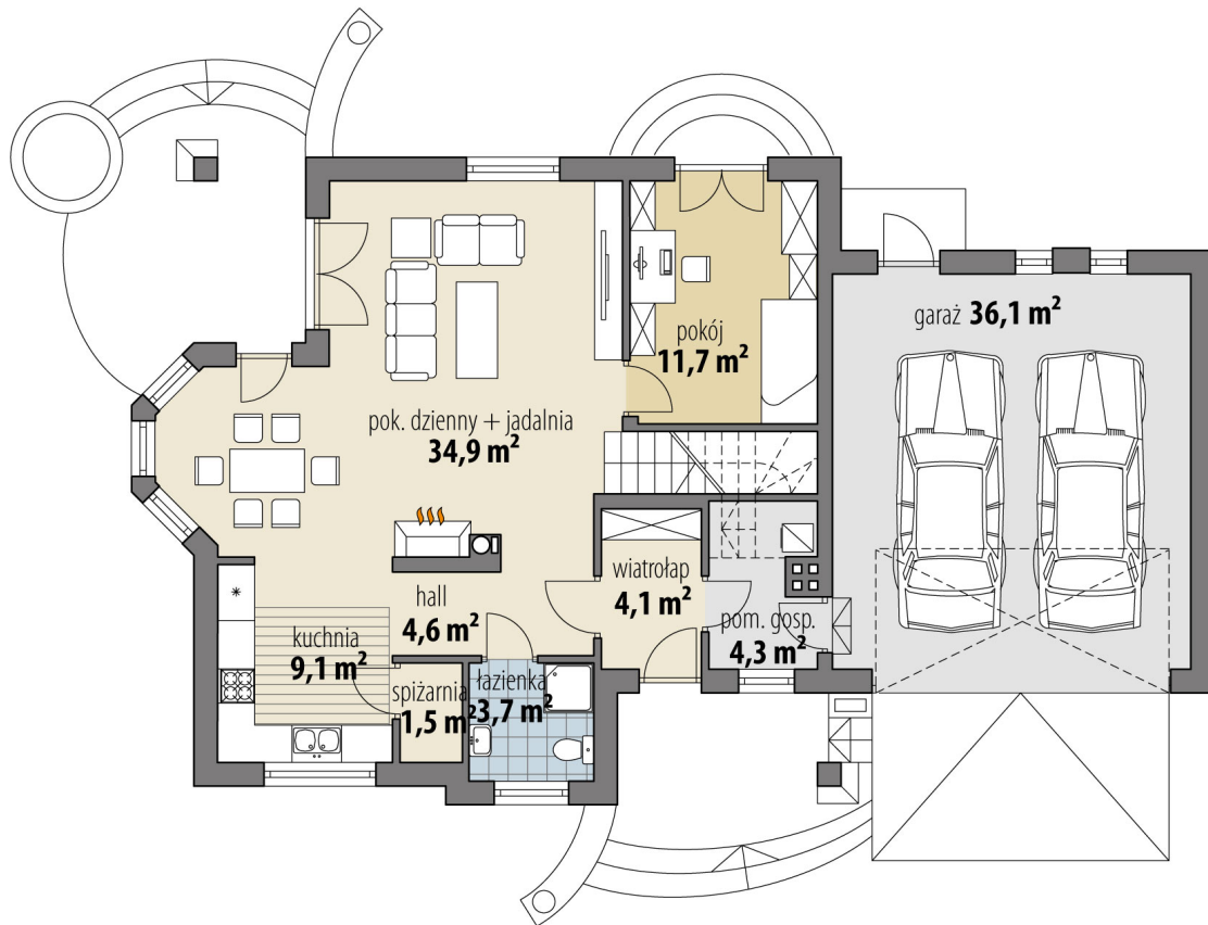
RZUT PARTER
