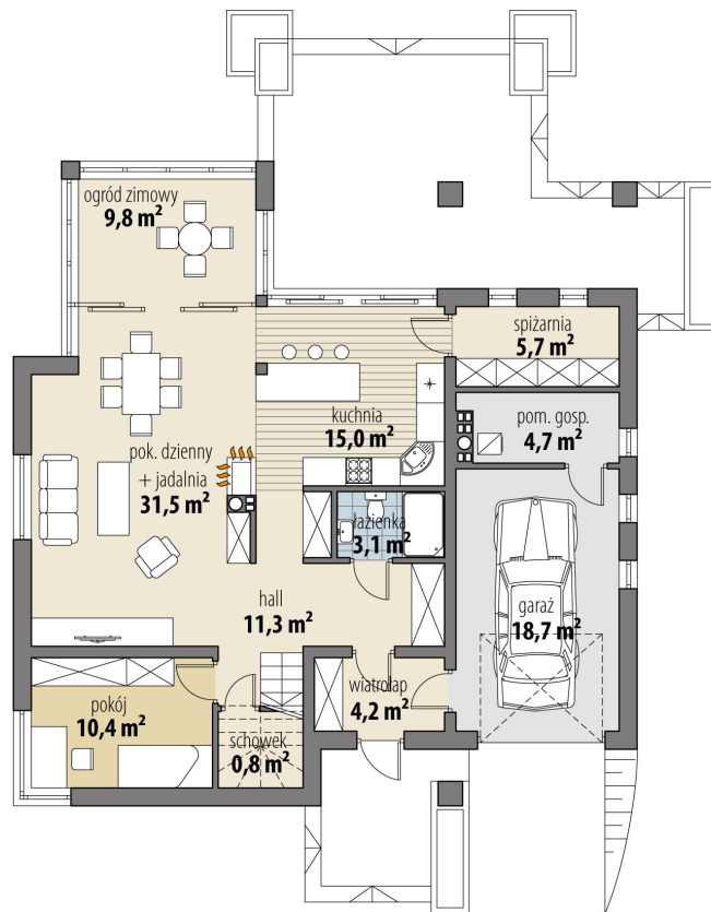
RZUT PARTER
