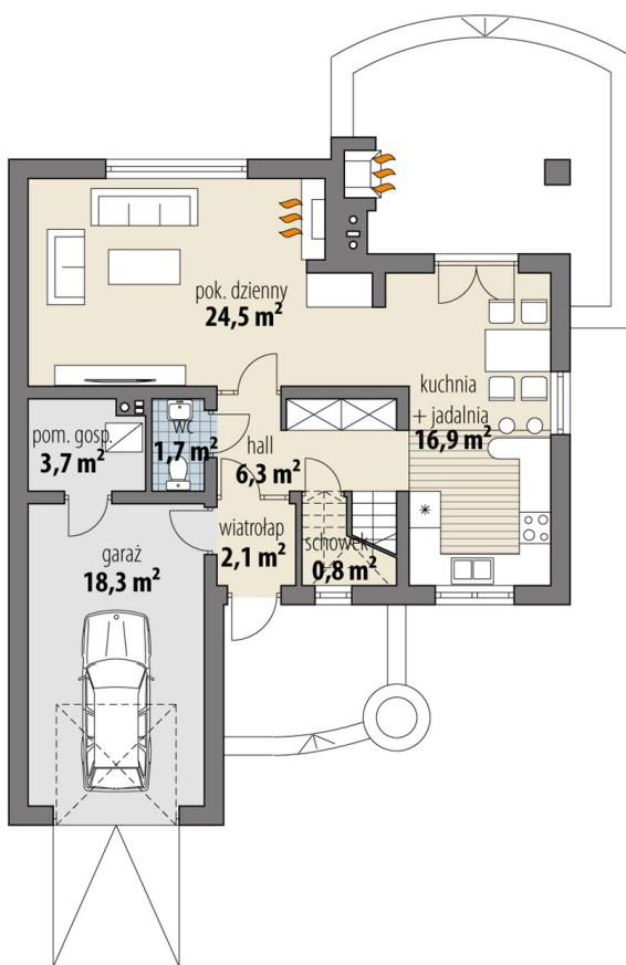
RZUT PARTER
