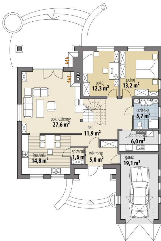
RZUT PARTER
