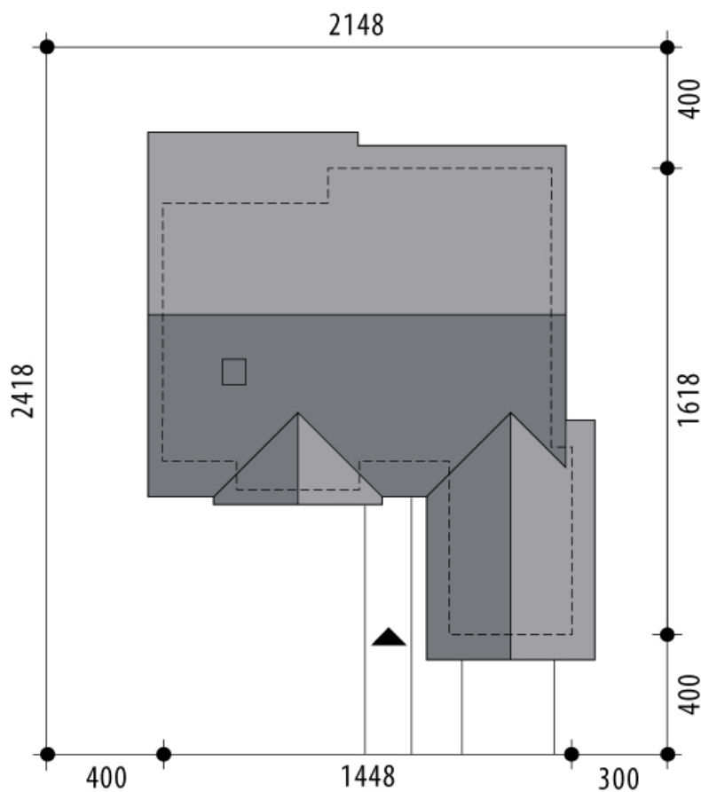
RZUT DZIAŁKI
