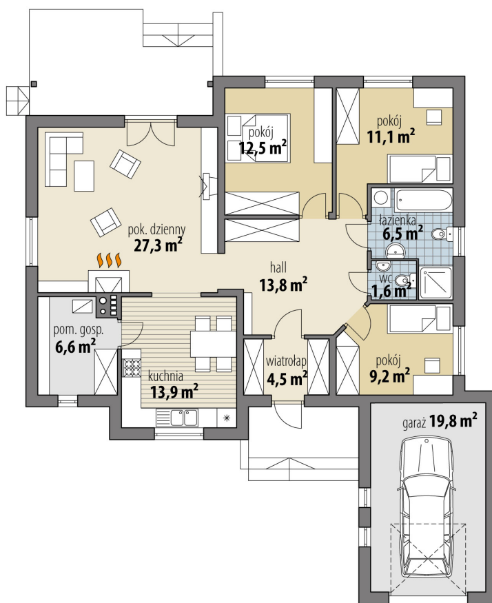
RZUT PARTER
