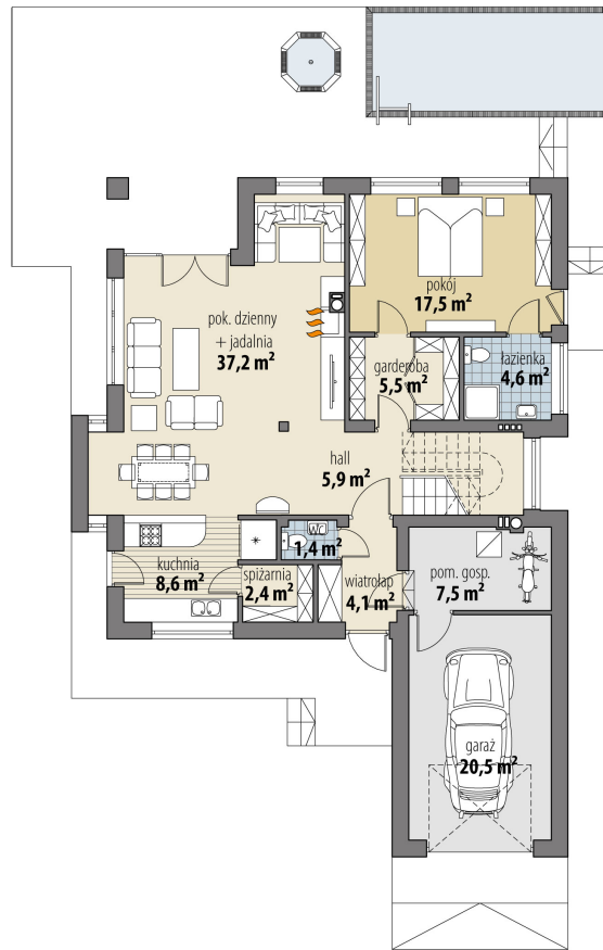
RZUT PARTER
