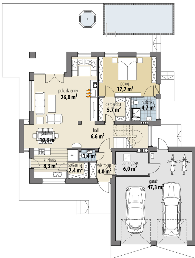
RZUT PARTER
