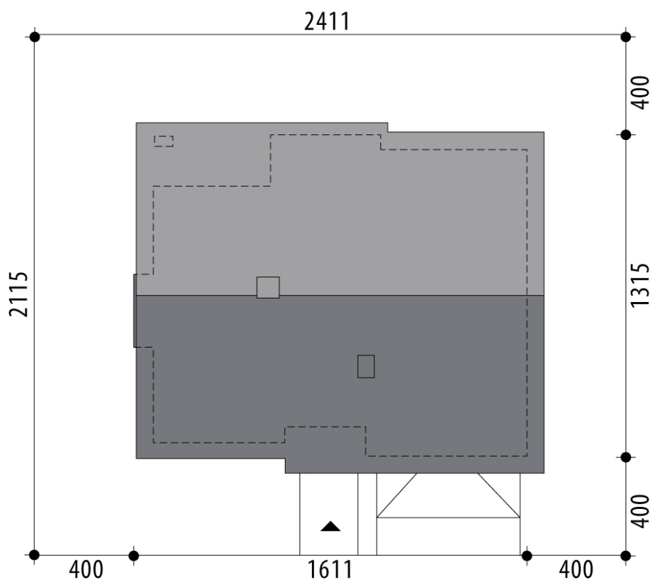
RZUT DZIAŁKI
