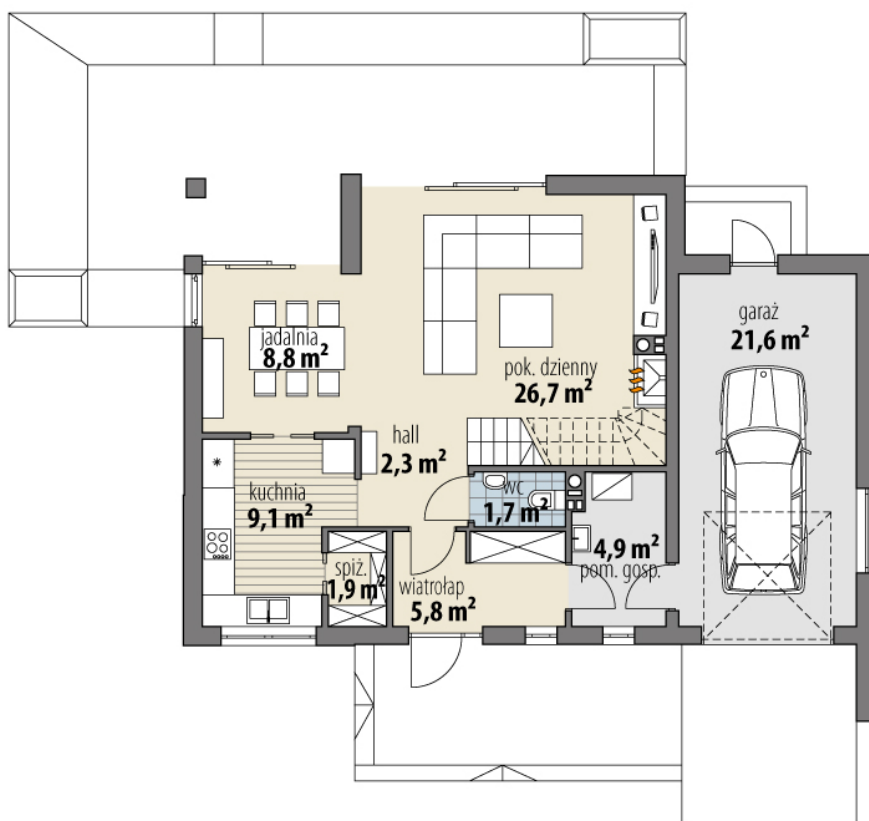
RZUT PARTER
