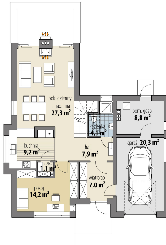
RZUT PARTER
