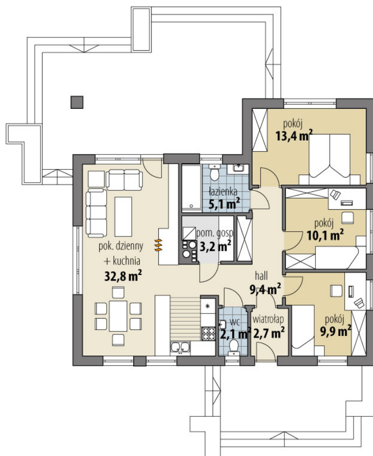
RZUT PARTER
