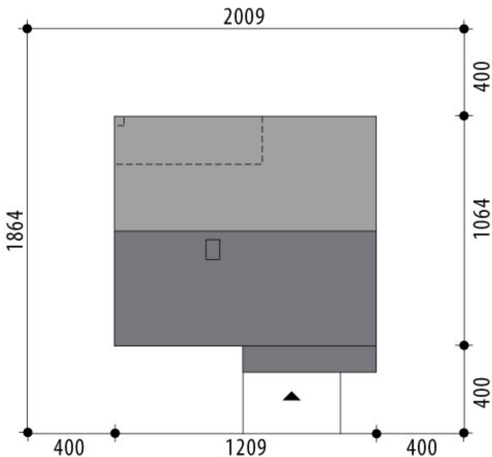
RZUT DZIAŁKI
