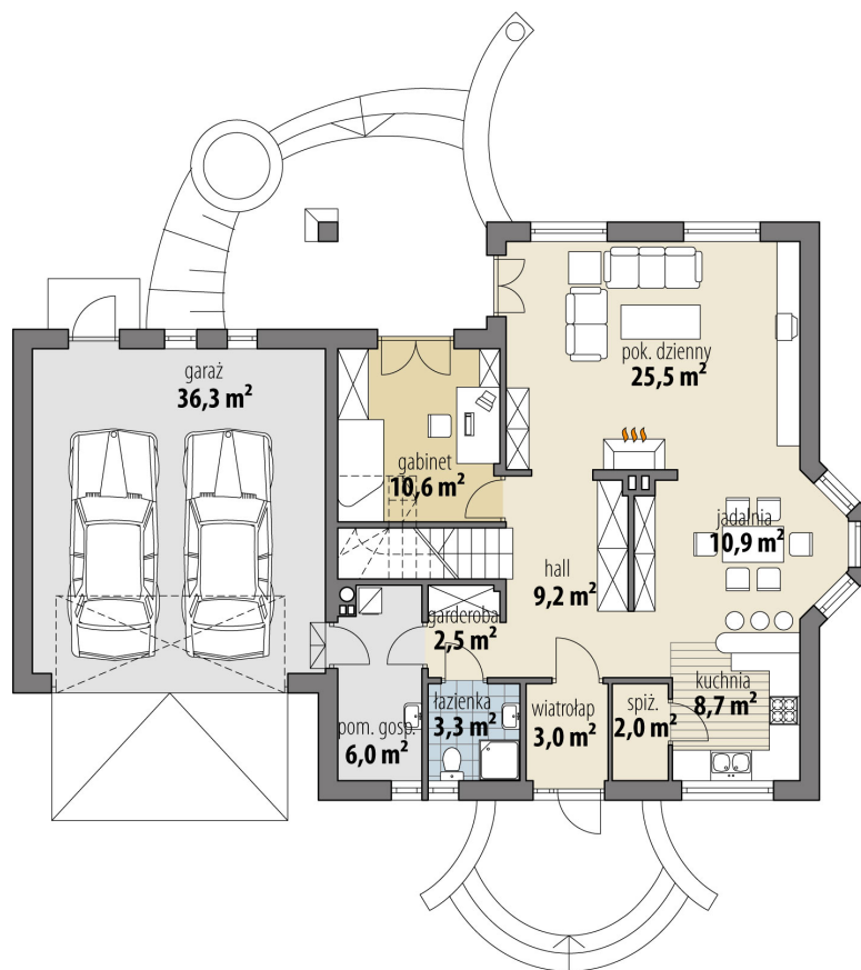
RZUT PARTER
