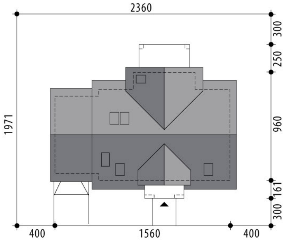
RZUT DZIAŁKI
