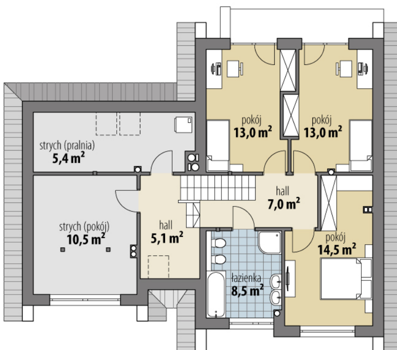
RZUT
