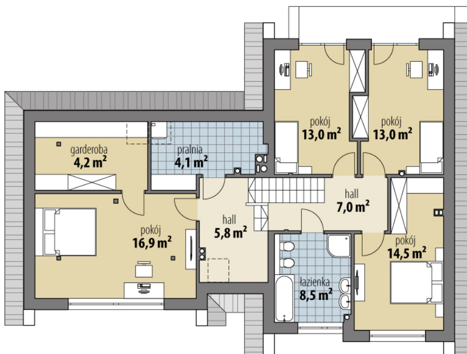
RZUT
