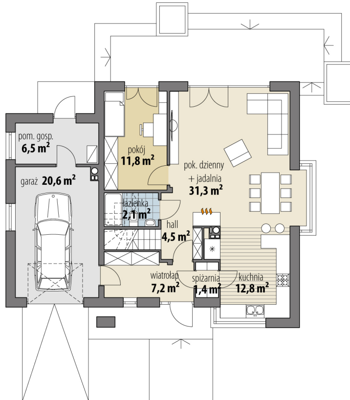
RZUT PARTER
