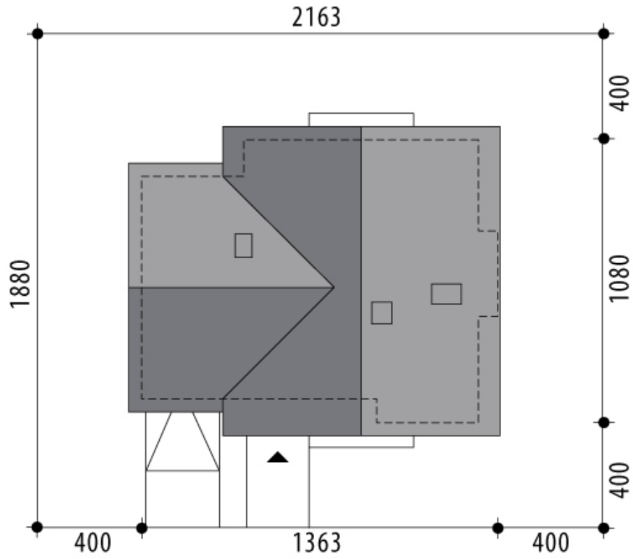
RZUT DZIAŁKI
