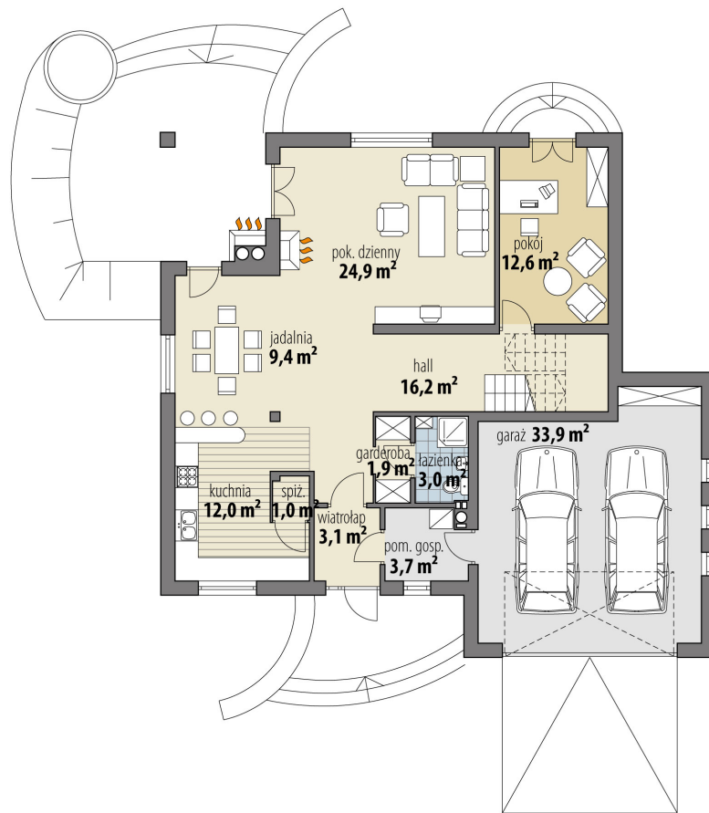
RZUT PARTER
