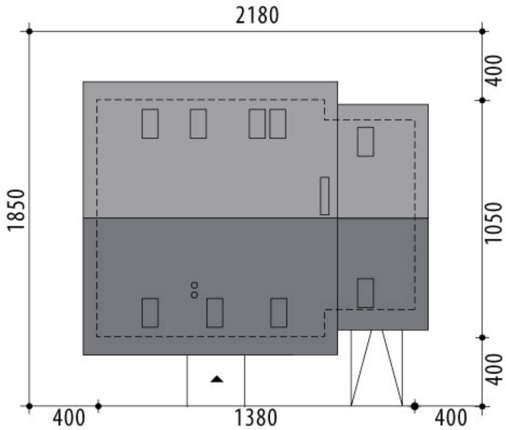
RZUT DZIAŁKI
