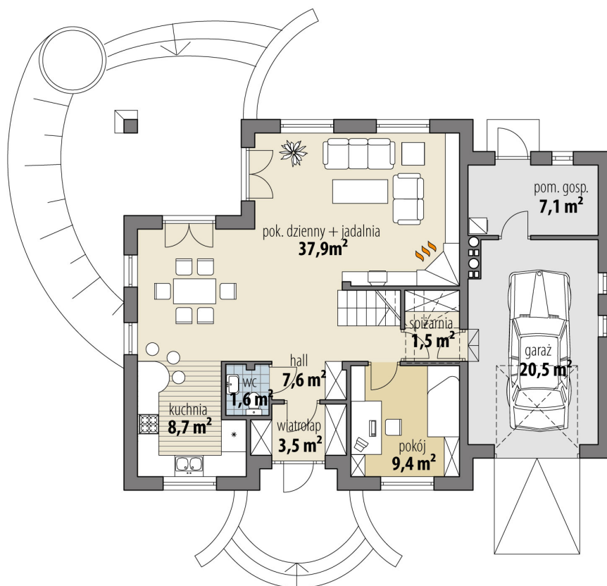
RZUT PARTER
