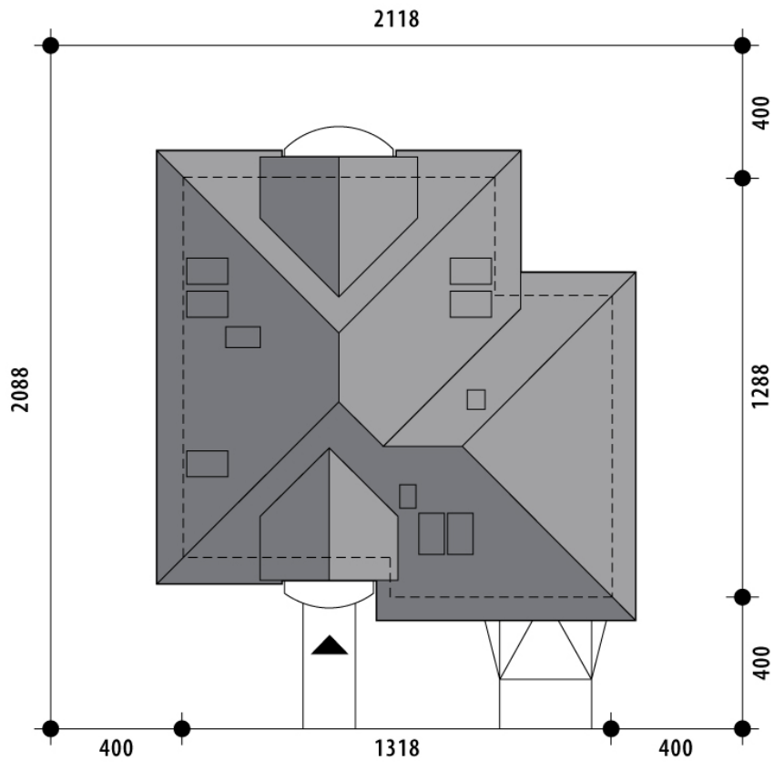
RZUT DZIAŁKI
