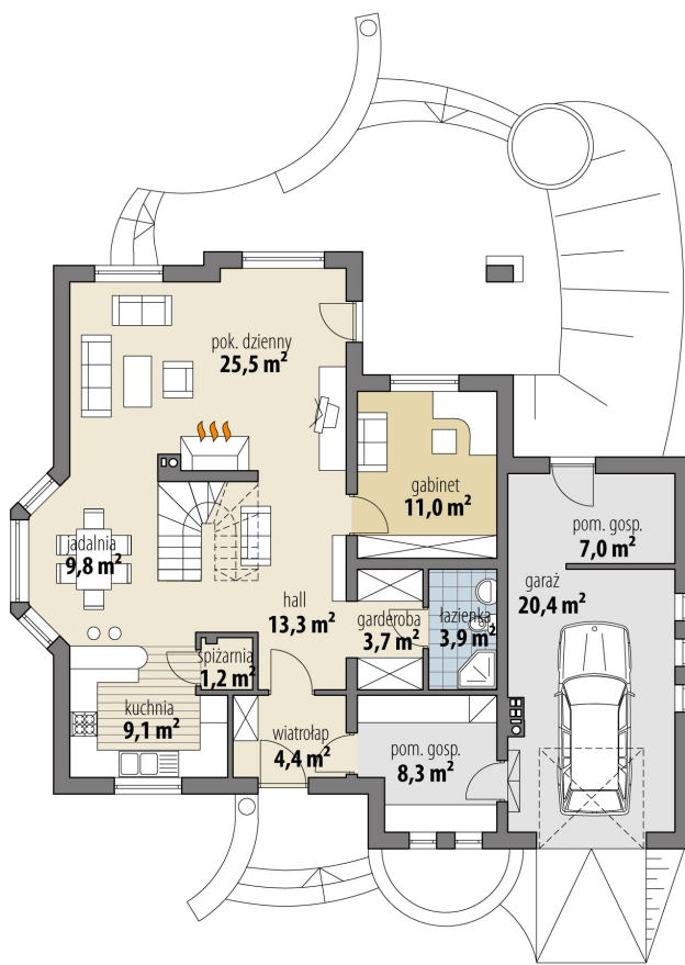
RZUT PARTER
