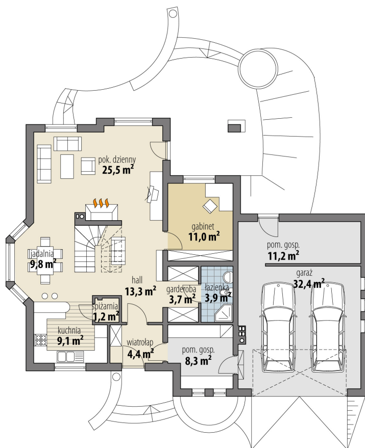
RZUT PARTER
