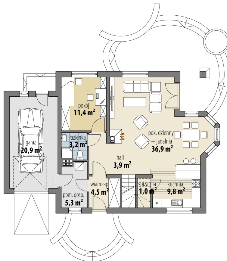
RZUT PARTER
