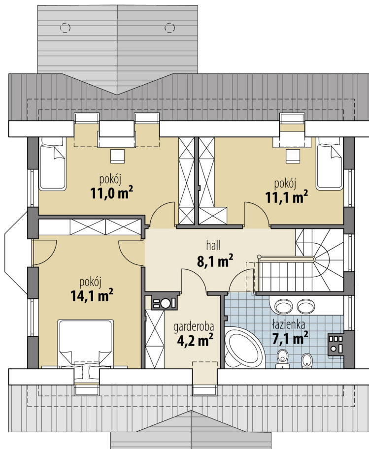
RZUT
