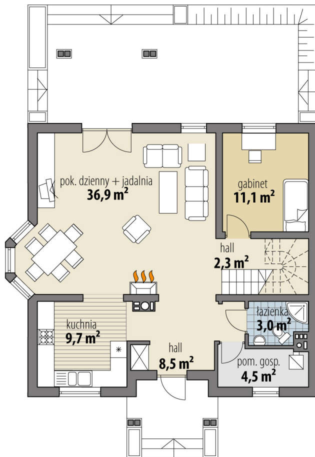
RZUT PARTER
