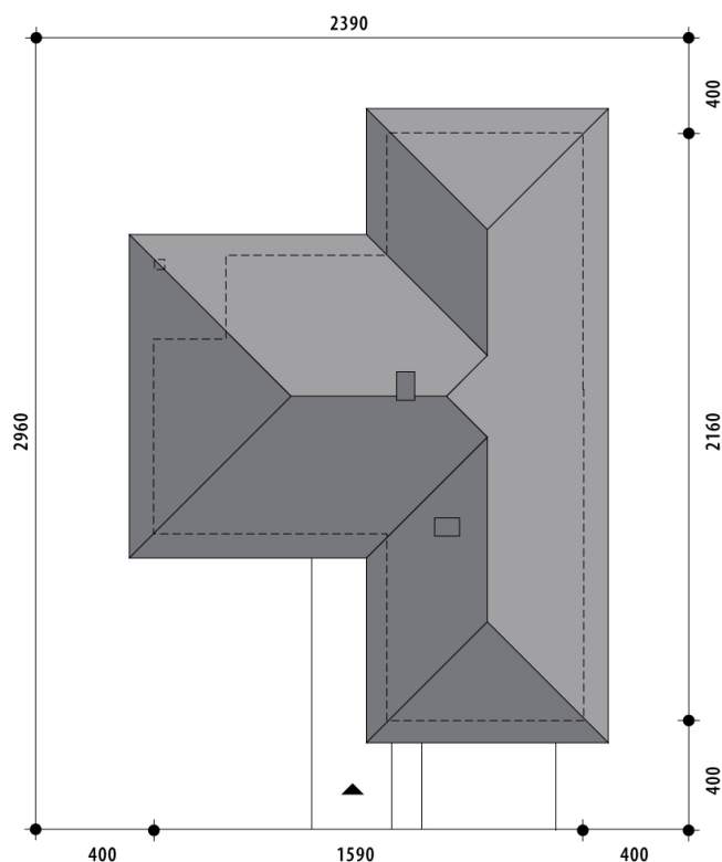
RZUT DZIAŁKI
