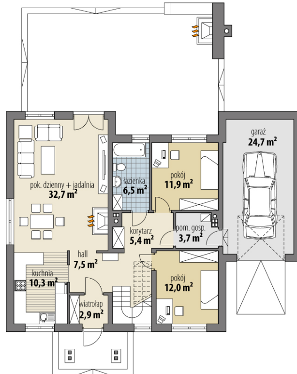
RZUT PARTER
