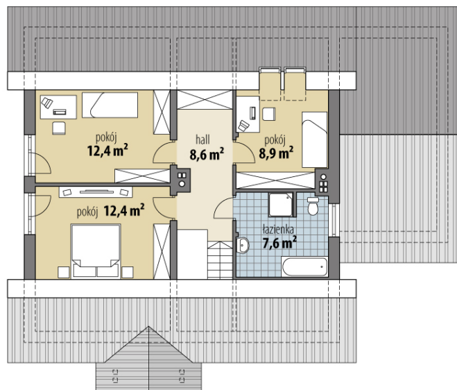
RZUT
