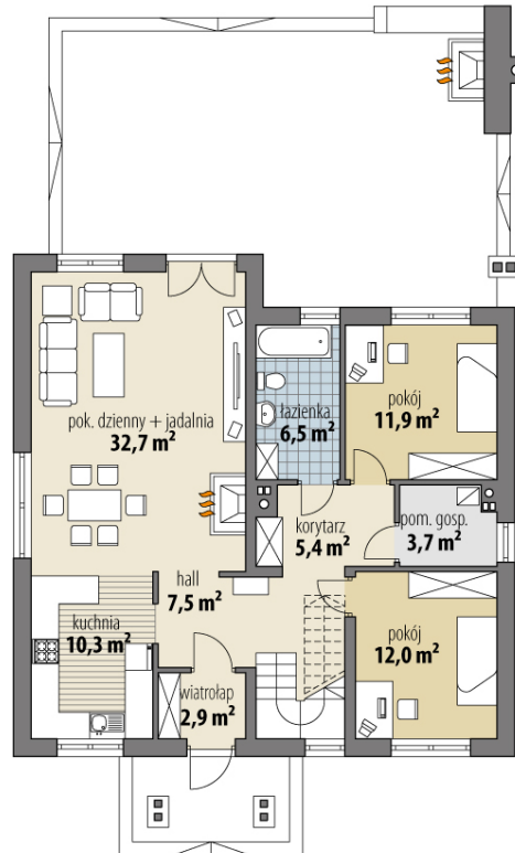
RZUT PARTER
