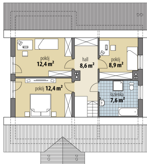
RZUT
