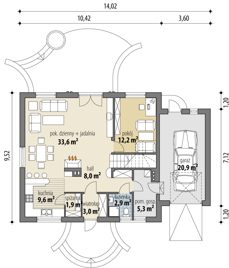
RZUT PARTER
