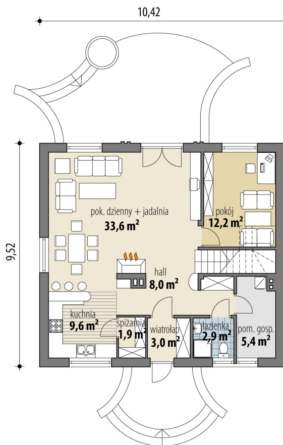
RZUT PARTER
