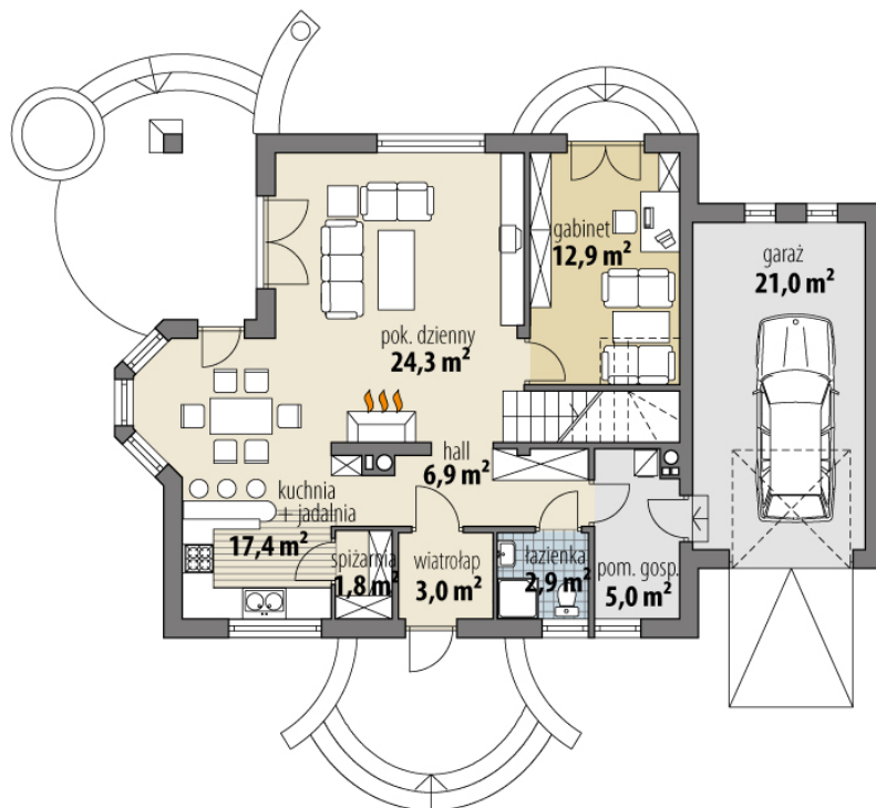
RZUT PARTER
