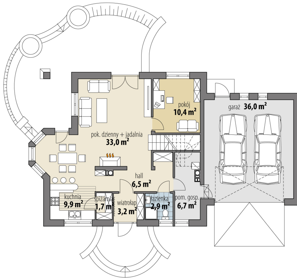
RZUT PARTER
