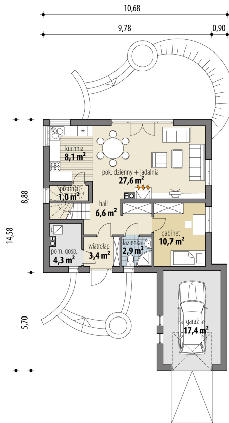
RZUT PARTER
