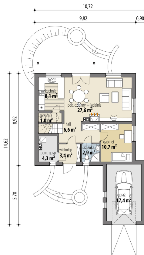
RZUT PARTER
