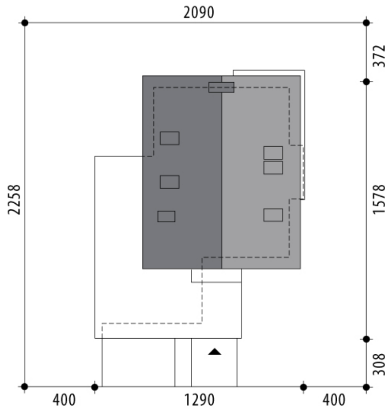
RZUT DZIAŁKI
