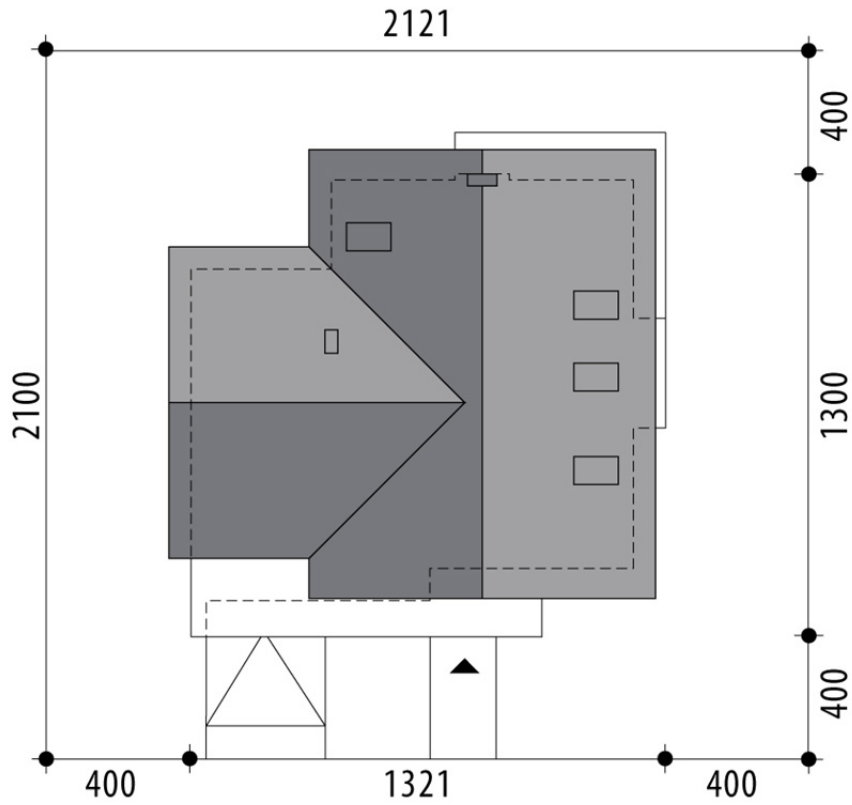
RZUT DZIAŁKI
